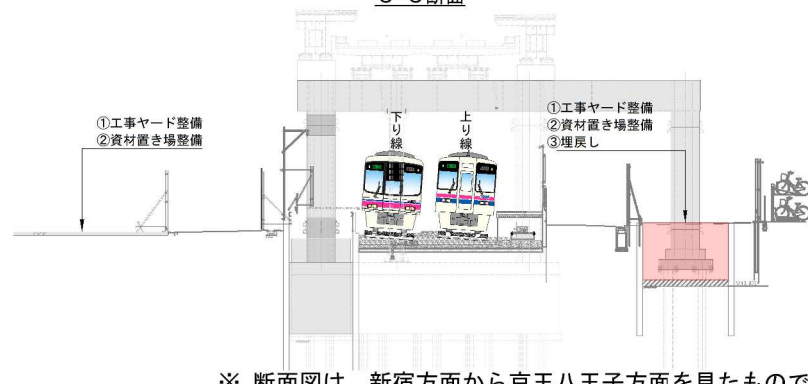
C-C断面
