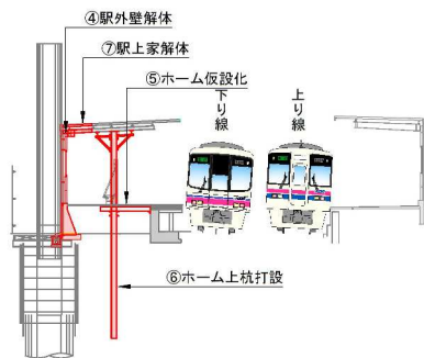
A-A断面
