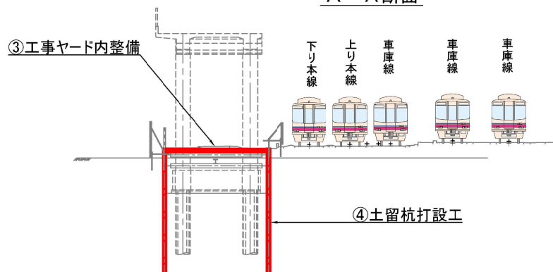
A-A 断面
