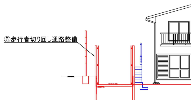
B-B 断面
