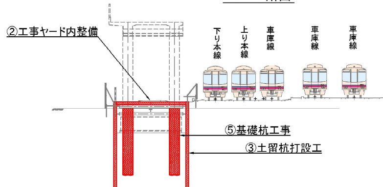
A-A 断面
