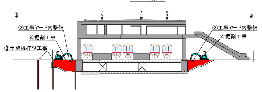
B-B 断面
