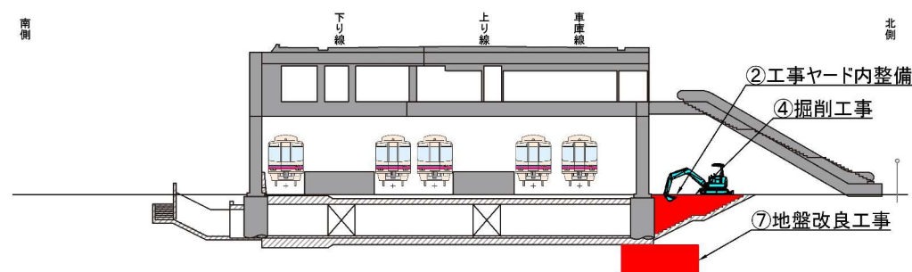
B-B 断面
