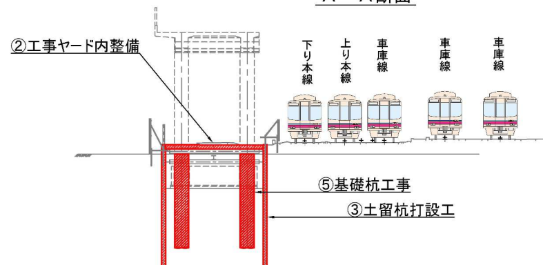
A-A 断面
