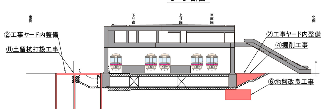
B-B断面
