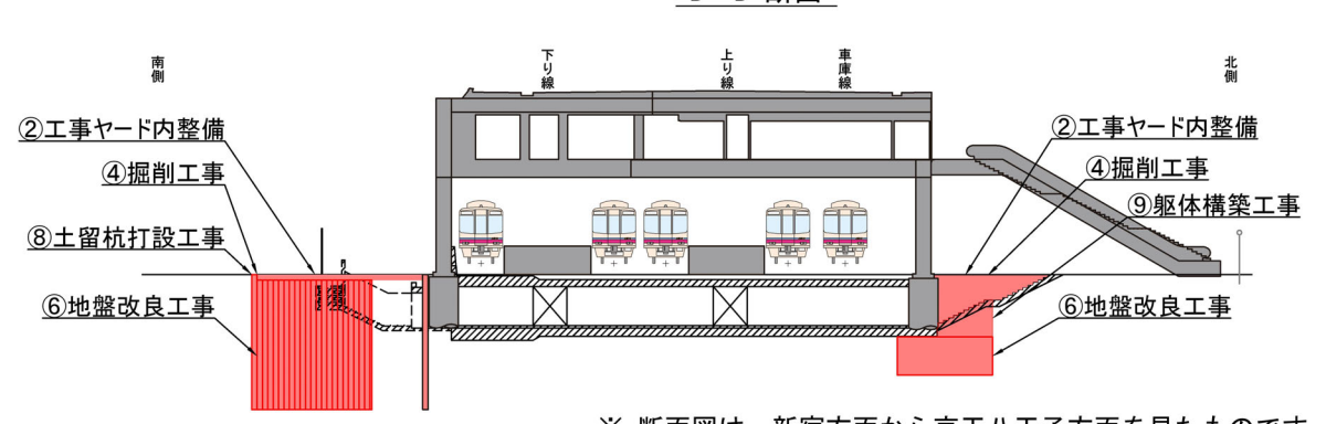
B-B断面
