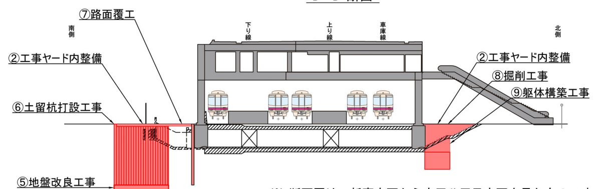
B-B断面
