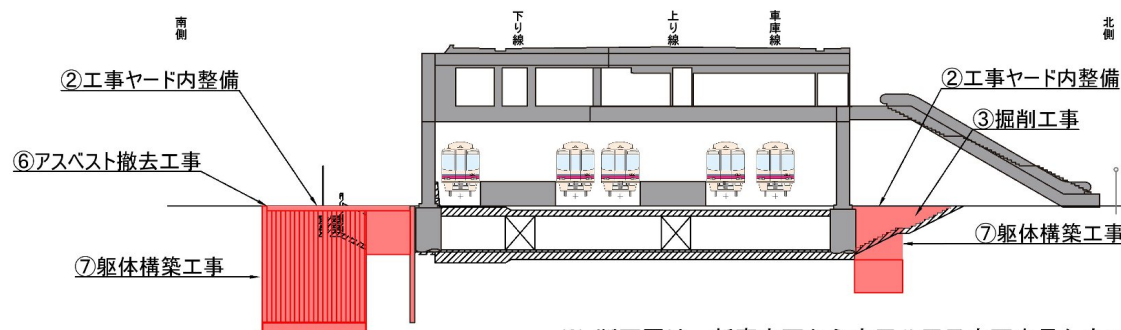
B-B断面
