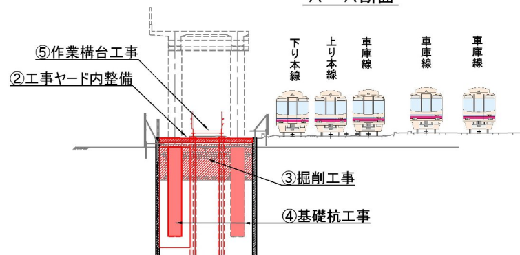
A-A断面
