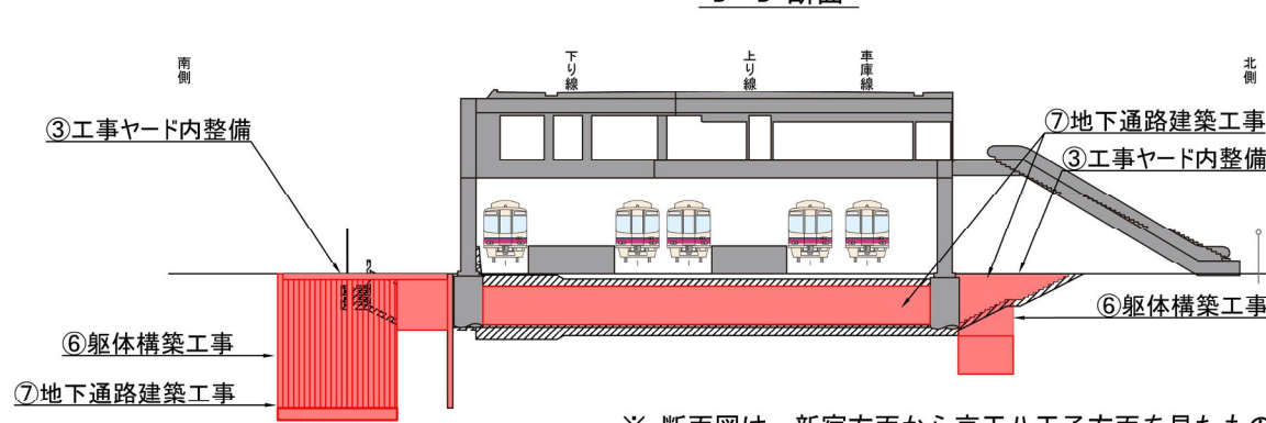
B-B断面
