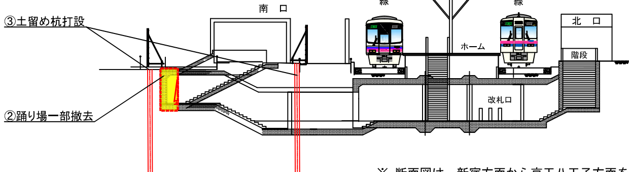
B-B断面図 (上北沢駅)
