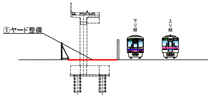
A-A断面図
