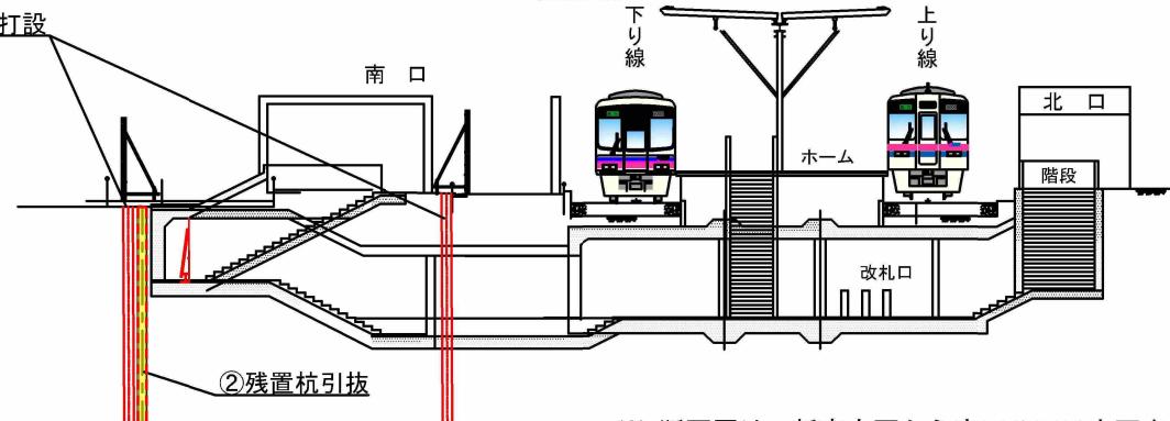
B-B断面図 (上北沢駅)
