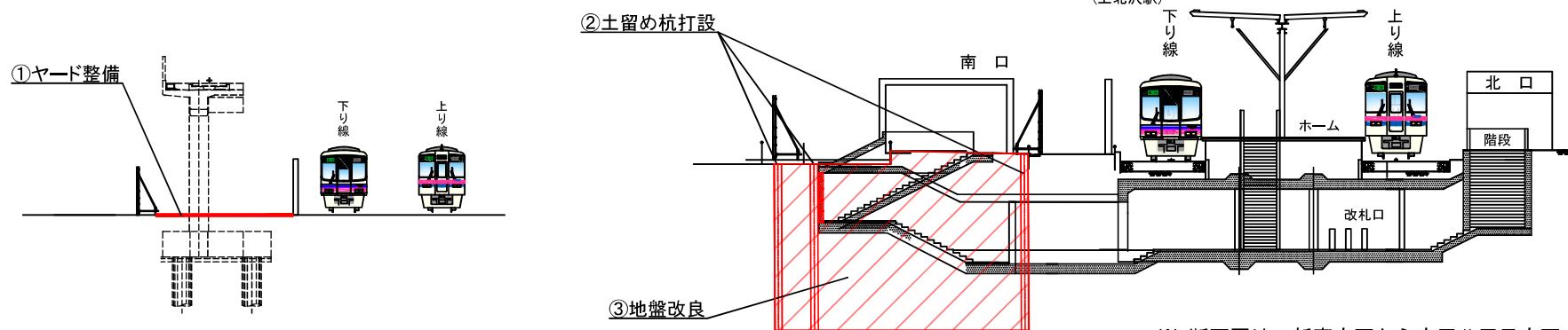
B-B断面図 (上北沢駅)
