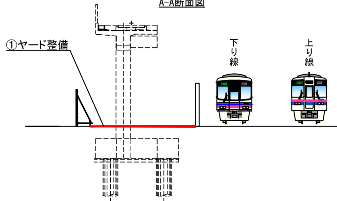
A-A断面図
