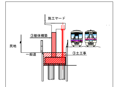
A-A 断面
