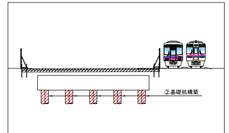
C - C 断面
