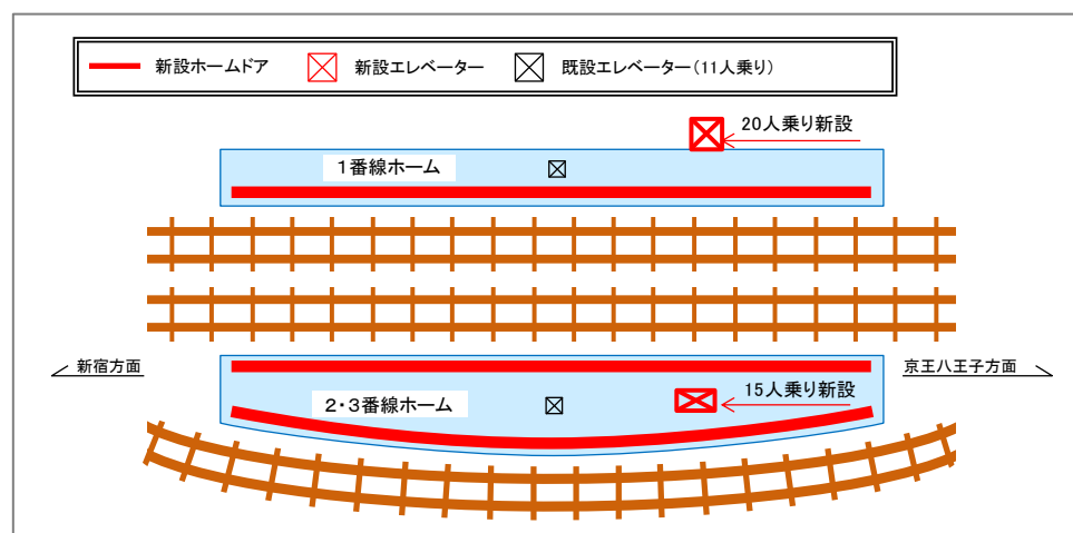
《新設設備計画図》
