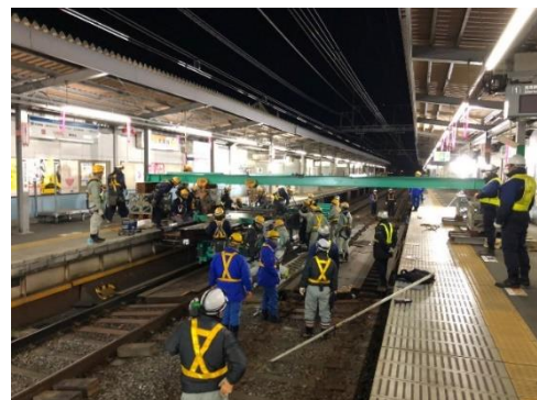
＜橋梁の架け替えの様子＞
